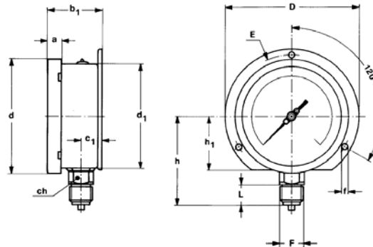
TIPO 3 Para montaje a pared. Con borde posterior y racord radial.
