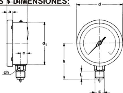
TIPO 1 Para montaje local directo. Con racord radial.
