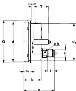
TIPO 6 Para montaje a panel. Con abrazadera y racord posterior.
