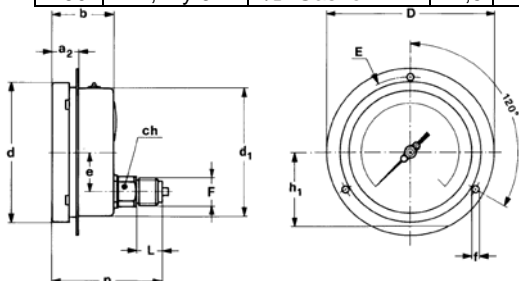
TIPO 4 Para montaje a panel. Con borde frontal y racord posterior.
