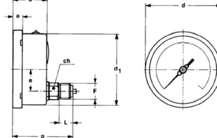
TIPO 2 Para montaje local directo. Con racord posterior.
